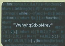
暗号技術
